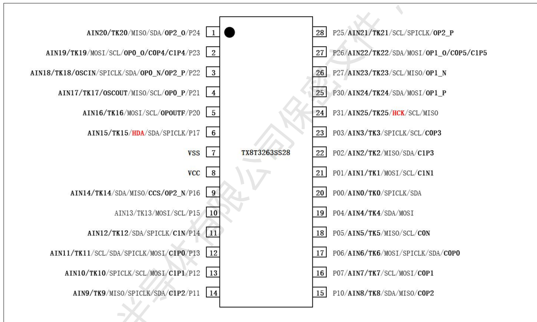
图 1 - TX8T3263SS28 (SSOP28) 封装图
